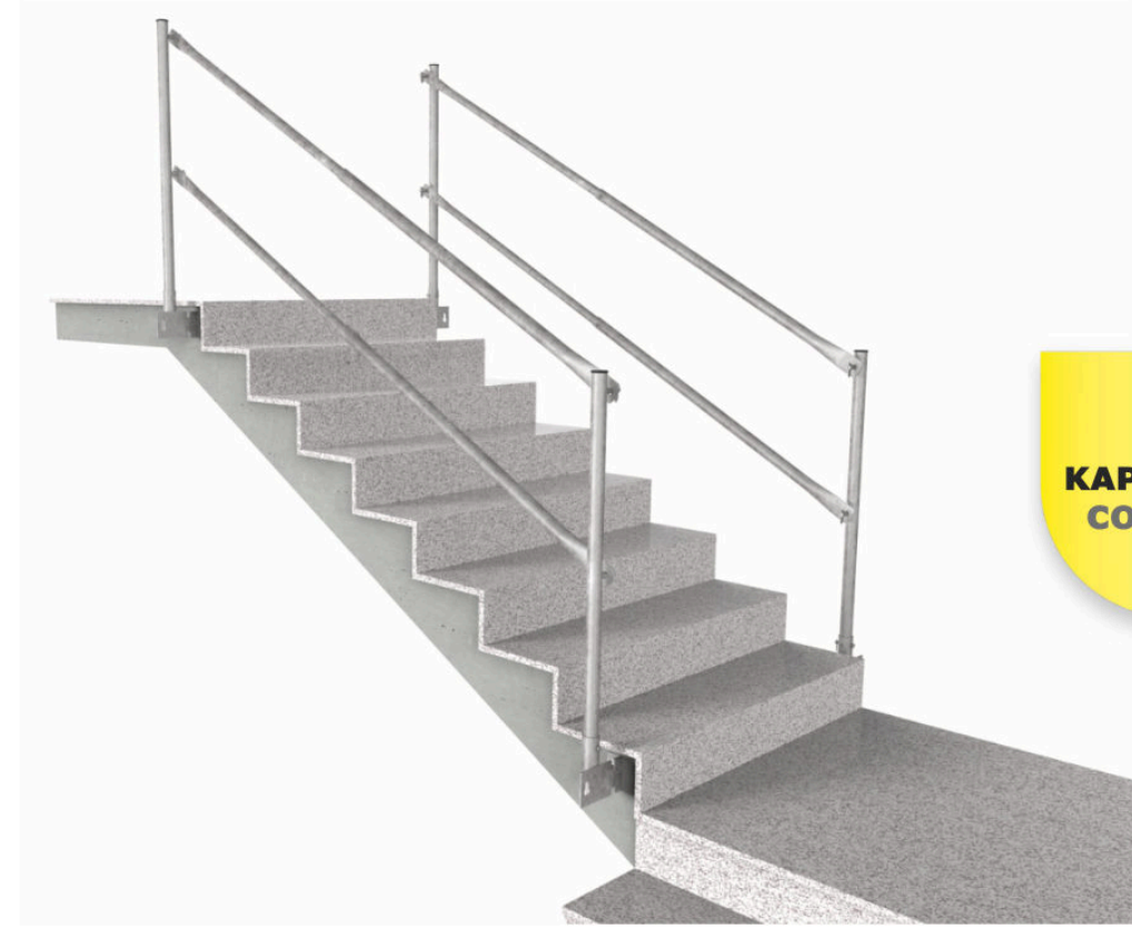
SAFETYBOARD Merdiven Alın Bağlantı Plakası Montajı SAFETYBOARD Guardrail Fixing Plate Assembly
