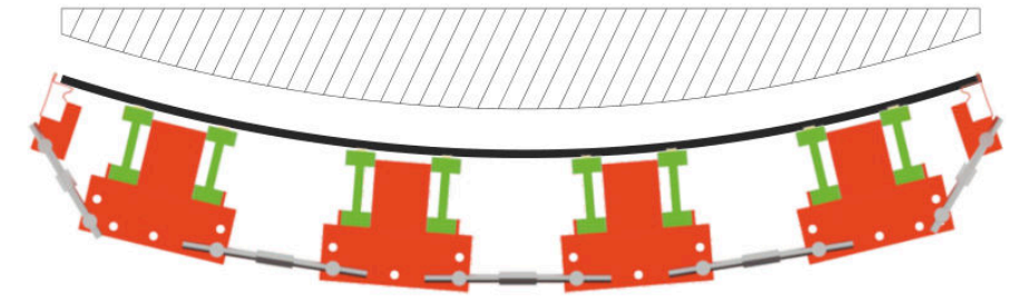
Adım 3 - Projeye göre şablon ile eğriliğin verilmesi Step 3 - Forming the curve according to the formwork design
