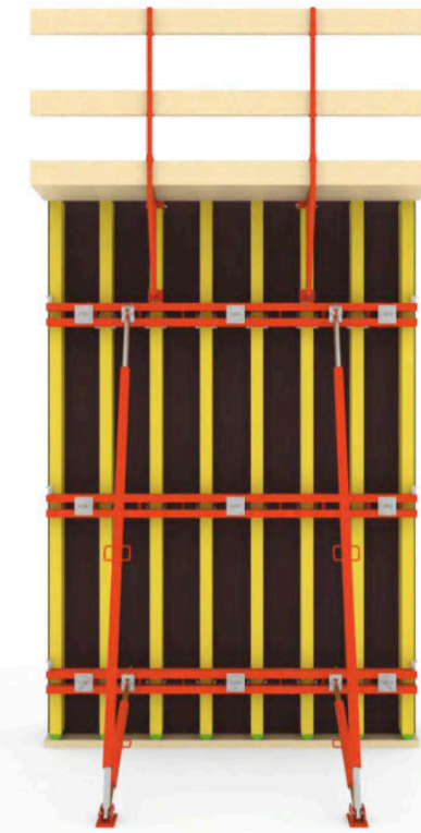
Timberform ahşap kirişli perde kalıbı tipik planı, görünüşü ve kesiti Timberform H20 Beam Formwork typical plan, view and section.
