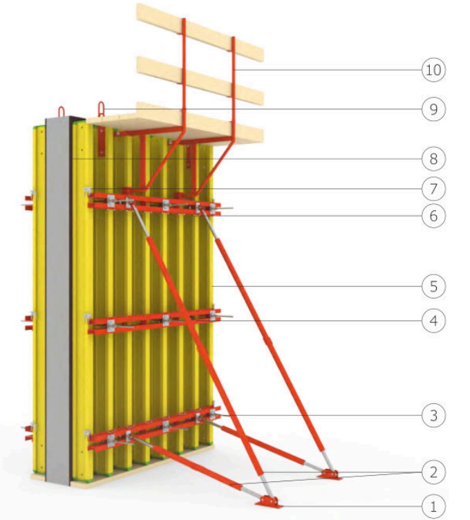
Timberform ahşap kirişli perde kalıbı tipik planı, görünüşü ve kesiti Timberform H20 Beam Formwork typical plan, view and section.
