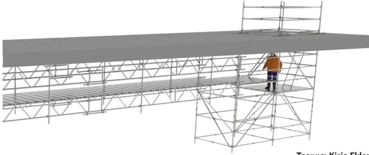
Taşıyıcı Kiriş Ekleme Elemanı Truss Beam Connection Component
